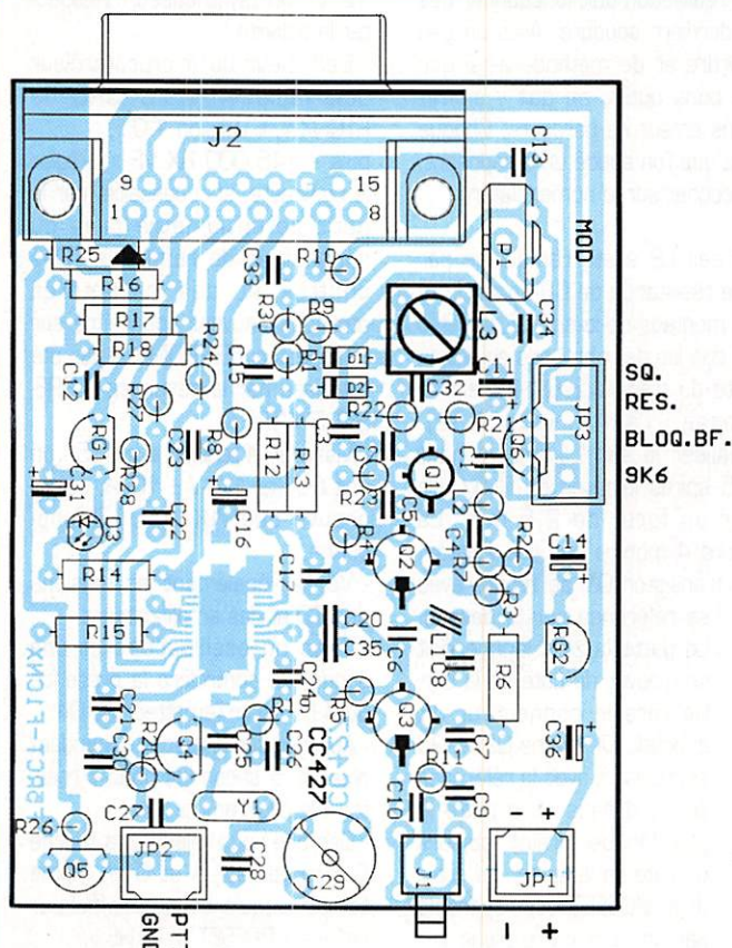
Implantation des composants.
