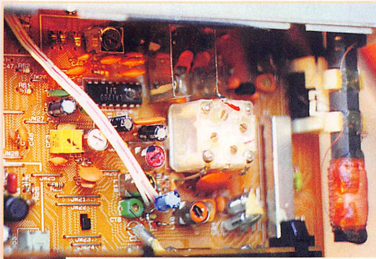
En jaune, les filtres céramiques du récepteur (455 kHz) sur lesquels on injecte le signal du BFO.
