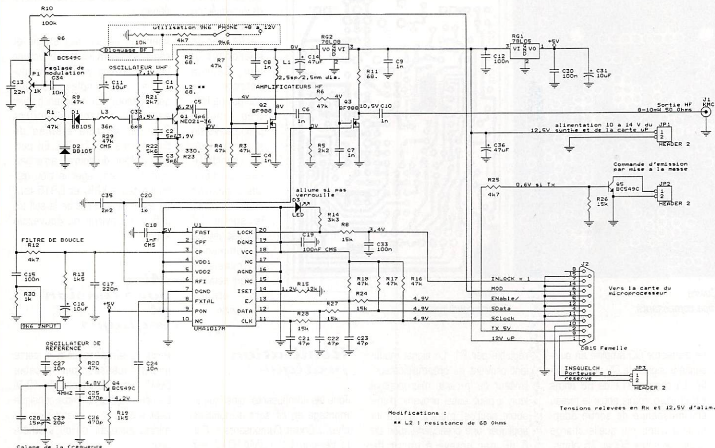
Schéma du synthétiseur UHF.
